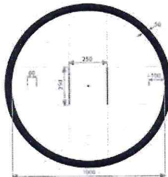
Рис. 1 «Игровое поле»
